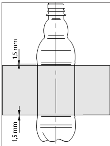
图 58: 重叠宽度
