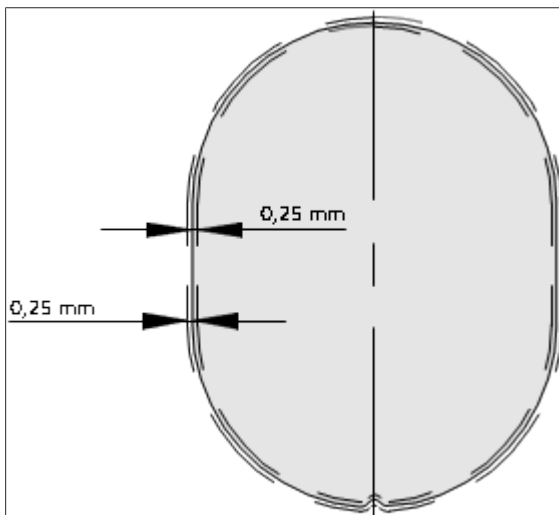
图 54: 标签公差
