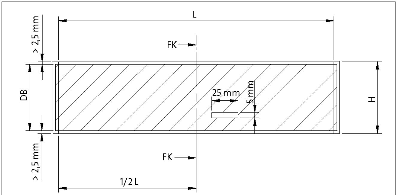
图 110: 标签尺寸
