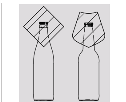
图 33: 尖角锡箔标： 在封盖处；下边缘有花边；在颈部区域重叠
