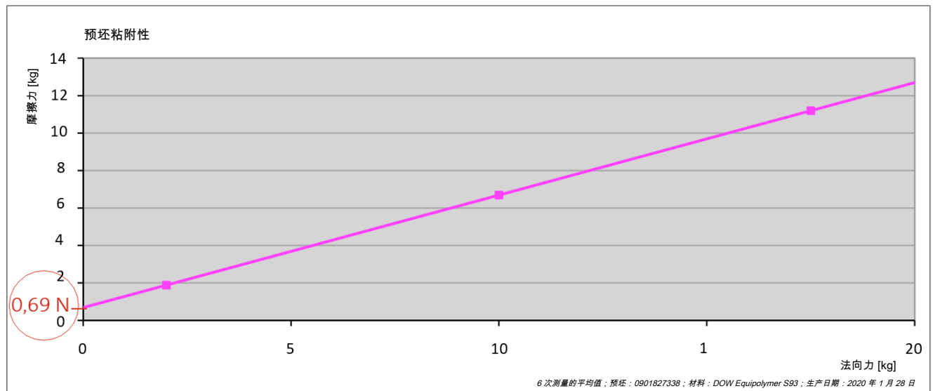
图 130: 粘附力随正向力的曲线图
