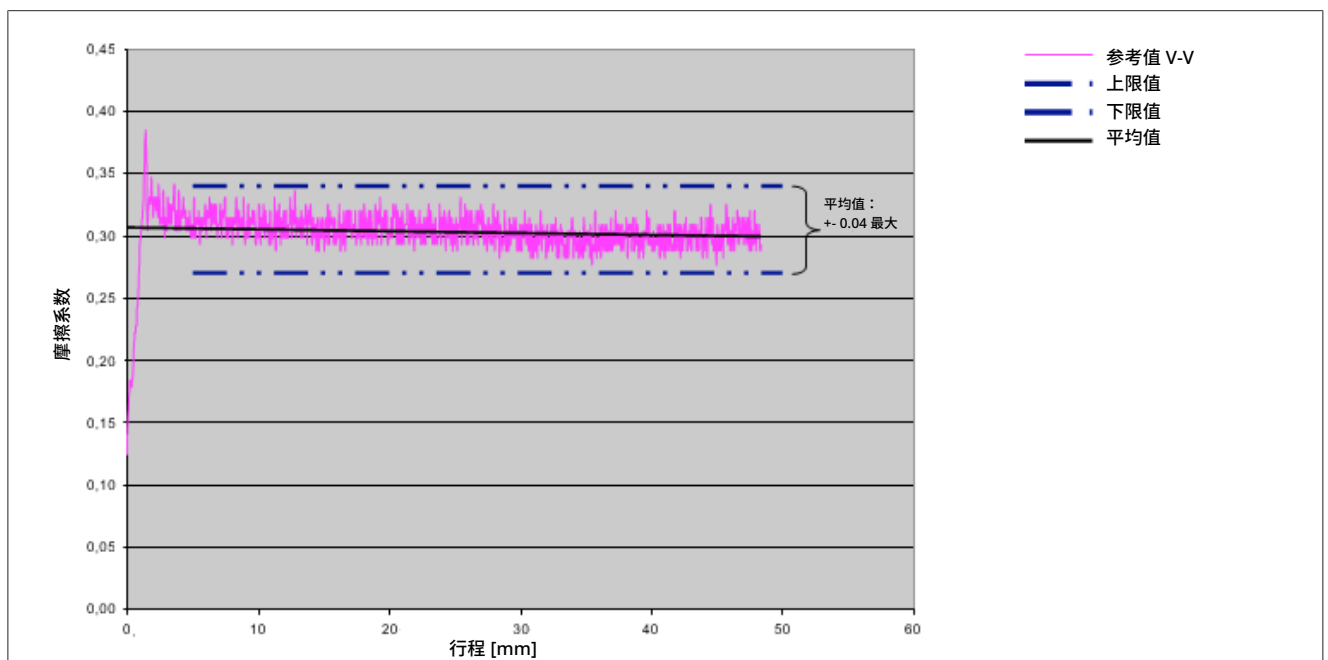
图 60: 标签的摩擦系数
