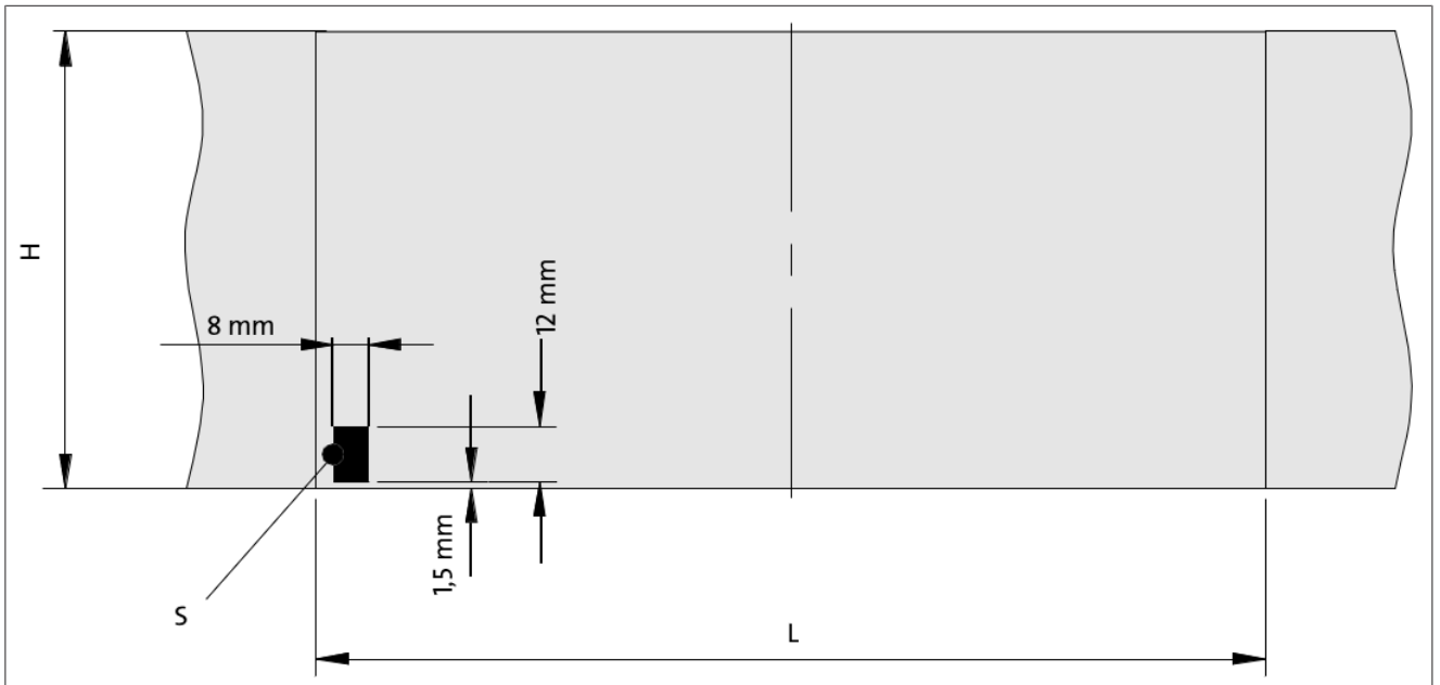
图 95: 荧光切割标记
