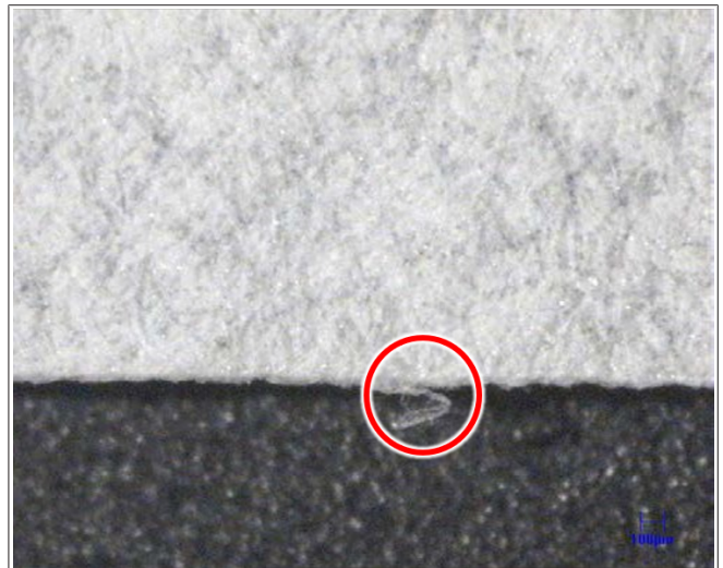
图 108: 切割边缘毛边
