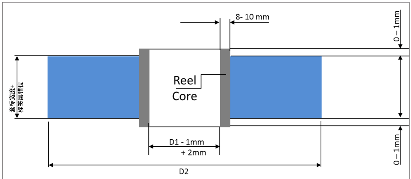
图 127: 套标标签的卷盘芯
