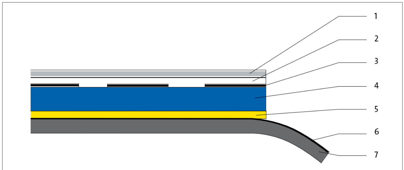
图 105: 材料结构
