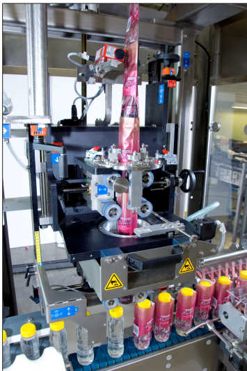
图 114: 切割标记的传感器扫描示例
