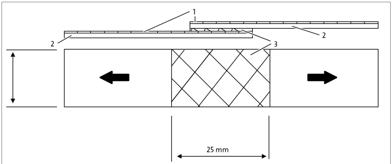
图 106: 标签的粘合
