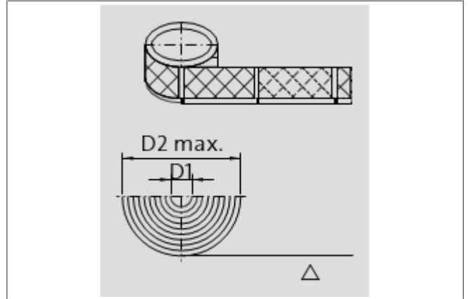
图 69: 机器运行方向从右到左的卷盘缠绕方向
