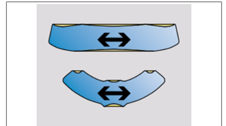
图 47: 正确的纤维走向
