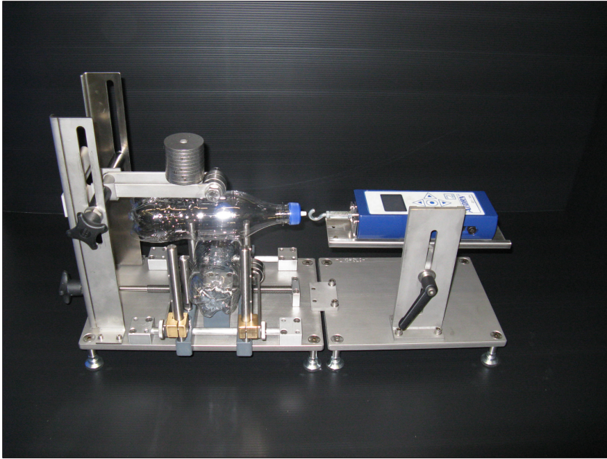
图 128: 瓶子粘附性测量装置
