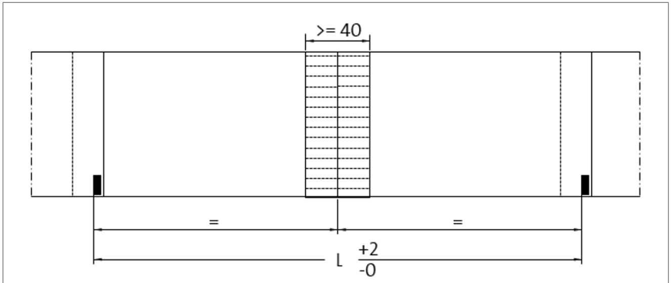
图 72: 适用于连续标签粘合的标签图样
