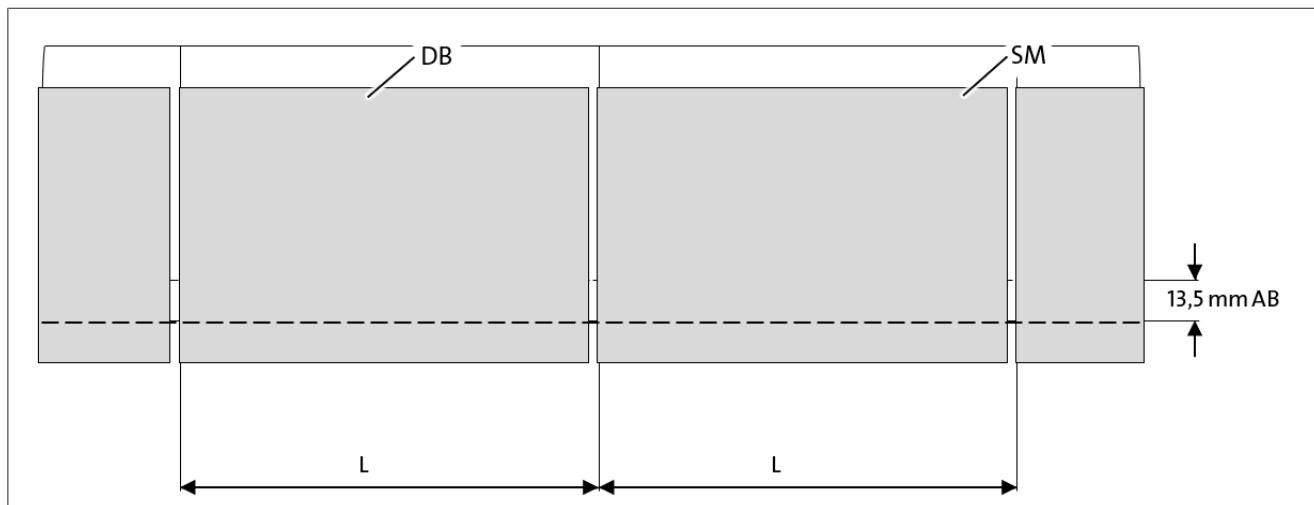
图 86: 带有透明切割标记的标签图样示例
