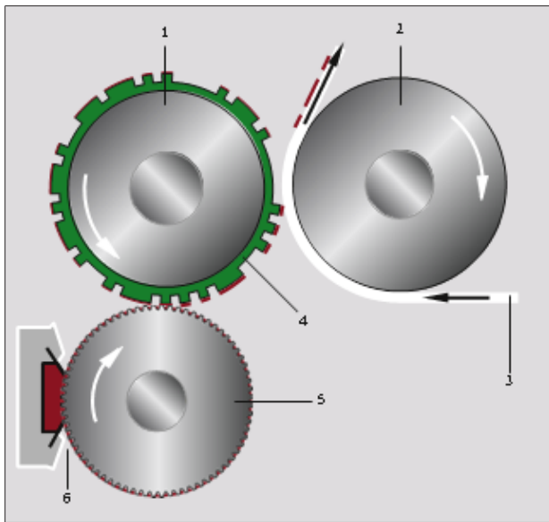
图8: 凸版印刷原理
