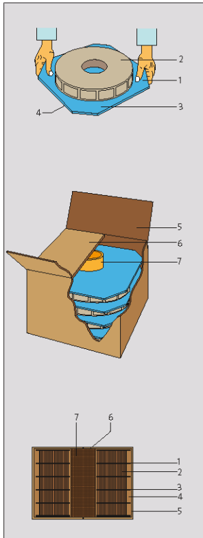
图 2: 卷盘标签的包装
