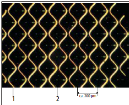
图 12: 机电雕刻网穴（最大雕刻深度）
