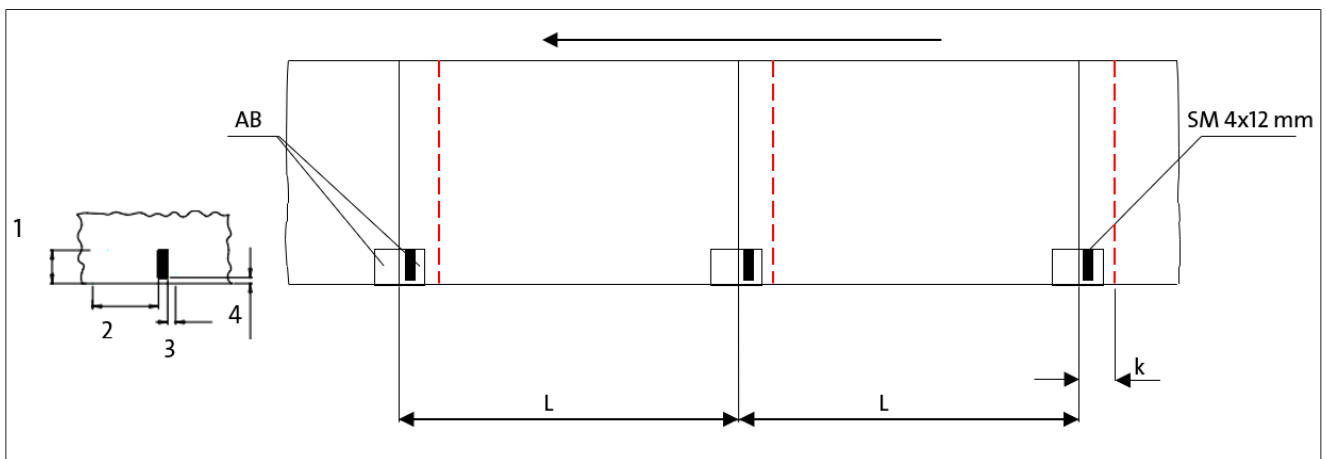
图 75: 通过一个窗口确定标签的扫描区域
