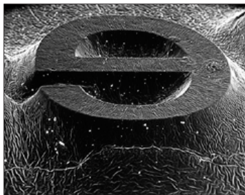
图 3: 凸版印刷印版的显微照片
