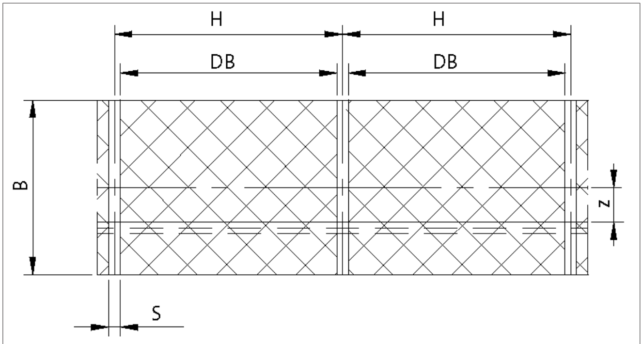
图 113: 图：标签尺寸
