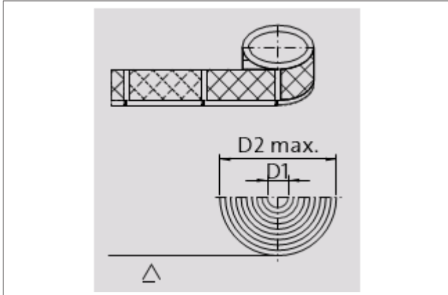
图 68: 机器运行方向从左到右的卷盘缠绕方向
