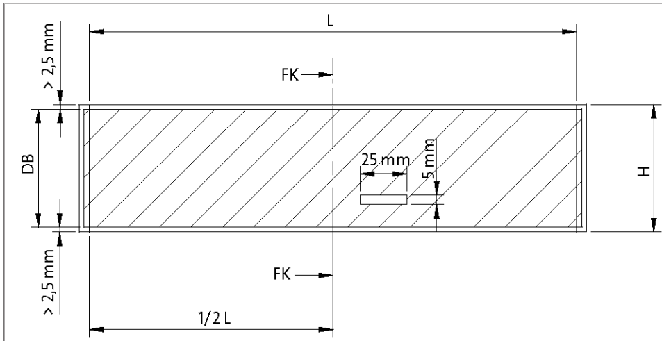
图 115: 用于套标标签切割标记几何形状的标签图样
