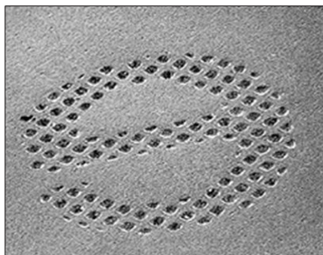
图 4: 凹版印刷印版的显微照片
