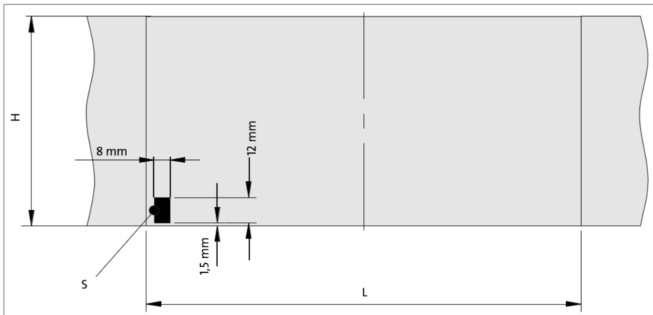
Рис. 95: Люминесцентная метка отрезания
