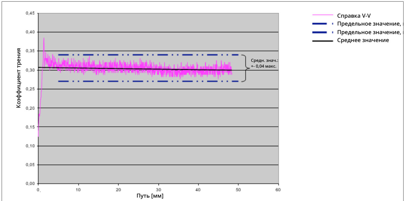
Рис. 60: Коэффициенты трения этикеток
