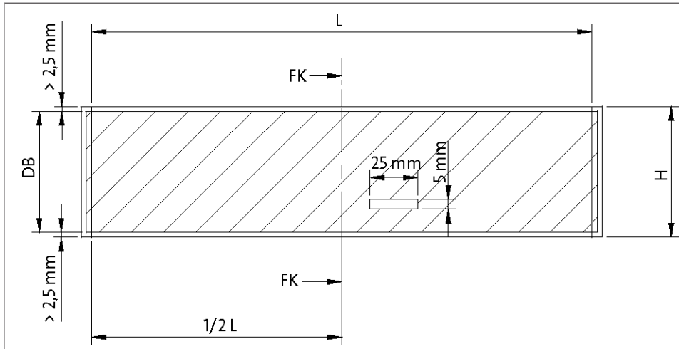
Рис. 115: Чертёж этикетки для геометрии метки отрезания рукавной Sleeve-этикетки
