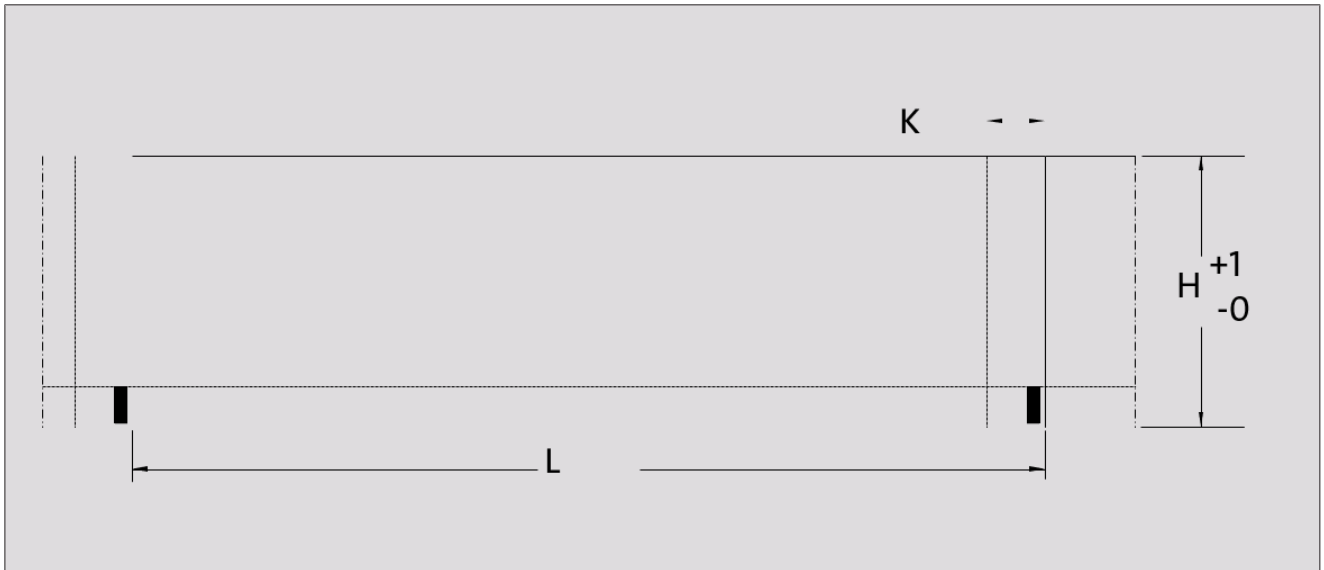
Рис. 59: Допуски на этикетки у этикеток в рулоне
