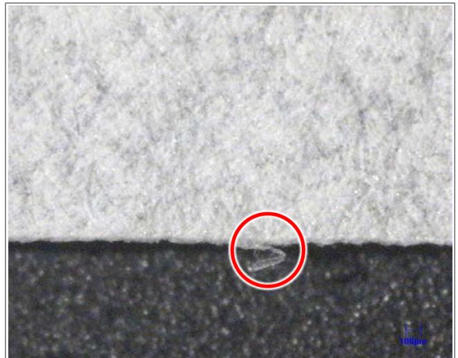
Рис. 66: Обрезанные края с бахромой
