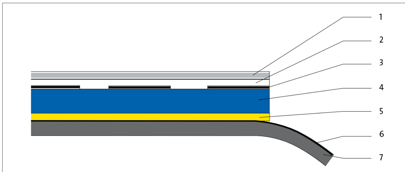
Рис. 105: Структура материалов
