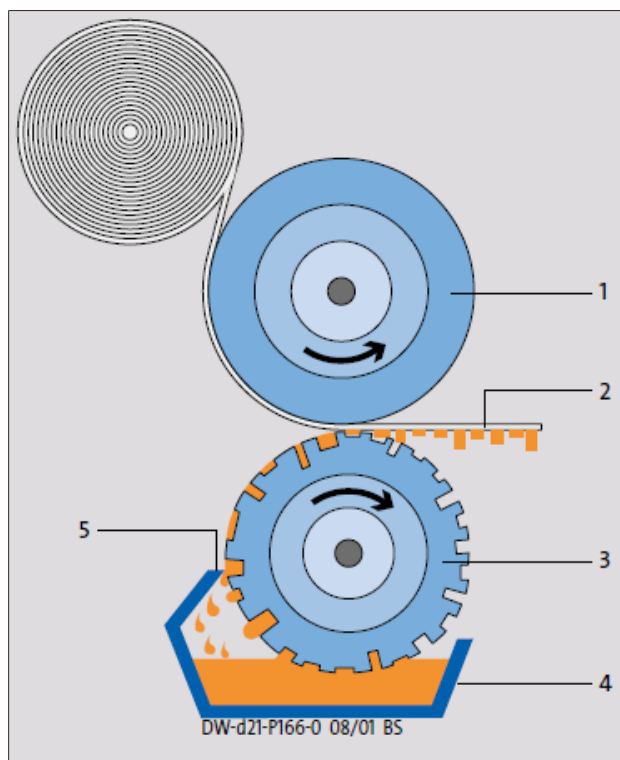
Рис. 11: Принцип глубокой печати
