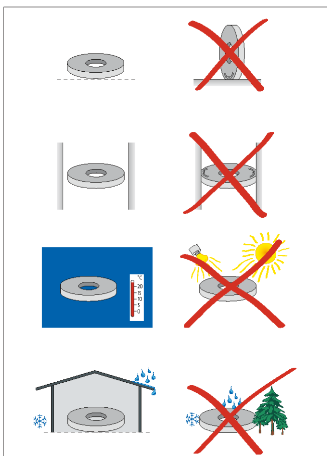
Рис. 1: Хранение непрерывной ленты этикеток
