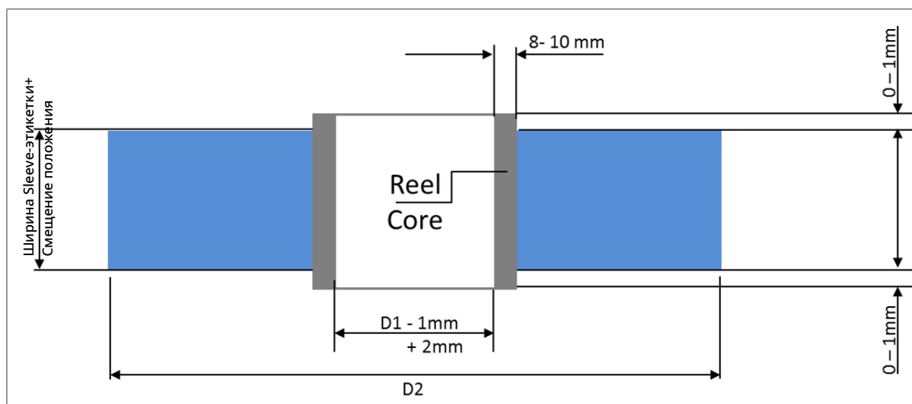
Рис. 127: Сердечник рулона у Sleeve-этикеток
