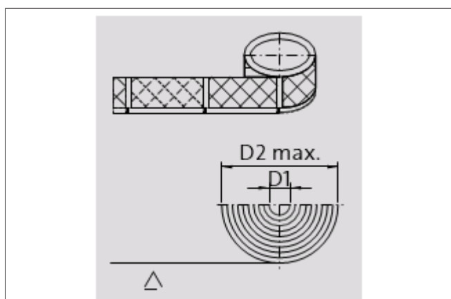
Рис. 68: Направление намотки рулона для направления движения в машине слева направо
