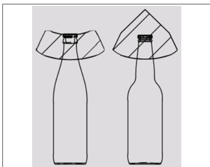
Рис. 32: Круговая станиолевая этикетка: выше пробки или на 2 мм ниже верхней кромки пробки; с закруглением по нижней кромке
