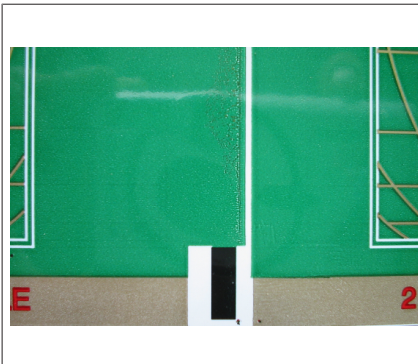
Рис. 91: Более одного цвета в зоне сканирования до и после метки отрезания и минимальный размер зоны сканирования не учтены.
