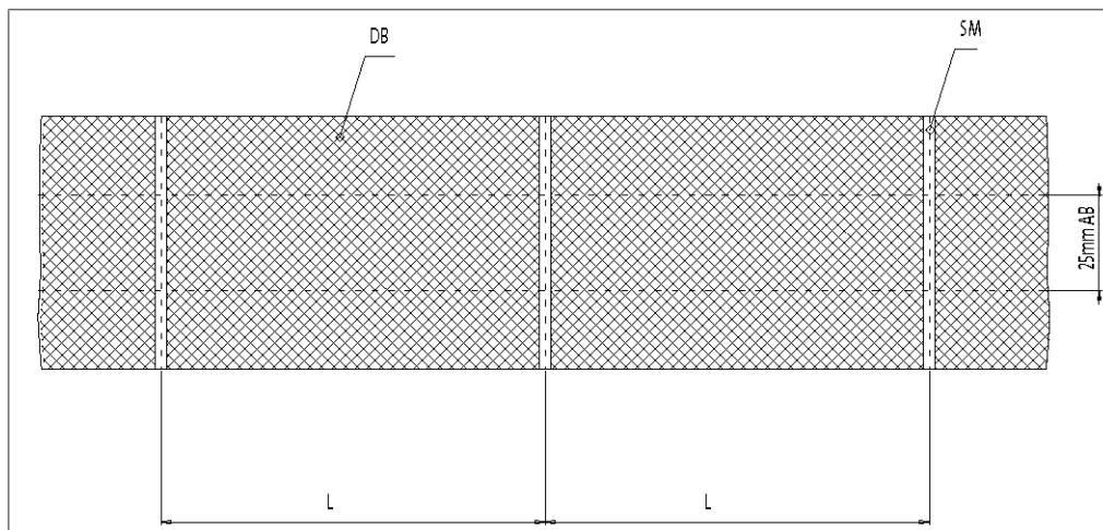
Рис. 121: Чертёж этикетки для геометрии метки отрезания с прозрачной меткой отрезания
