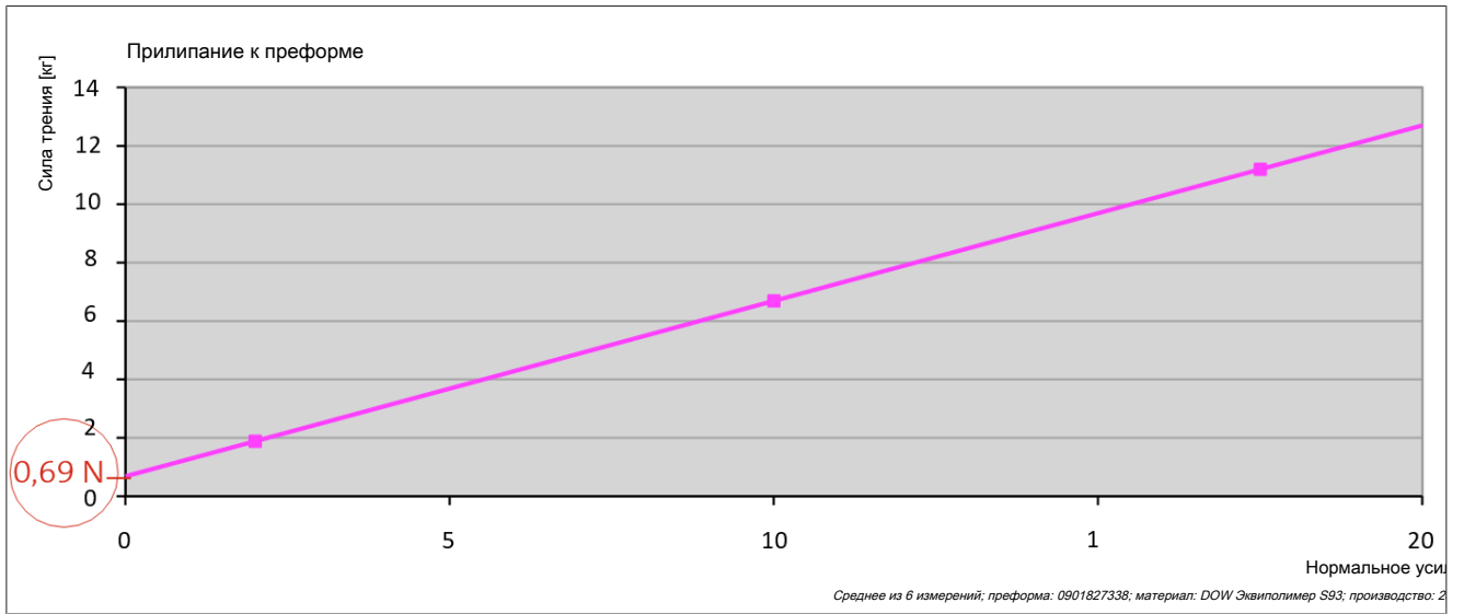
Рис. 130: Изменение силы сцепления по отношению к нормальному усилию
