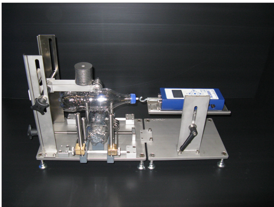
Рис. 128: Прибор измерения показателей прилипания бутылок
