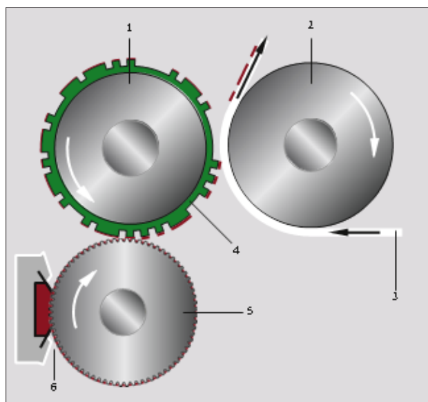
Рис. 8: Принцип печати высокого давления
