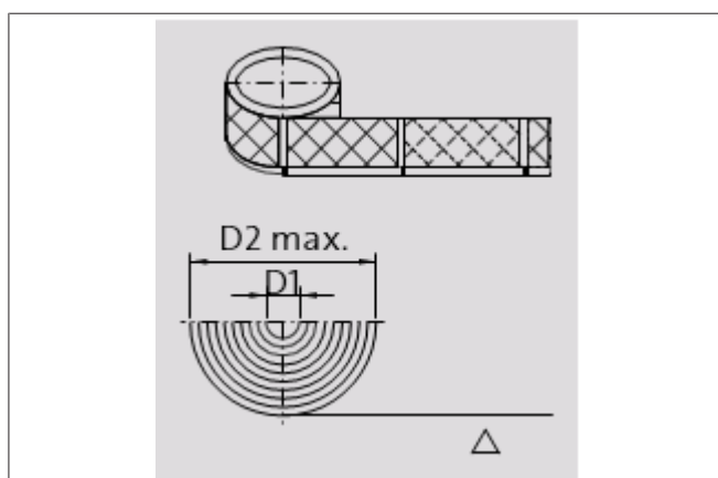
Рис. 69: Направление намотки рулона для направления движения в машине справа налево
