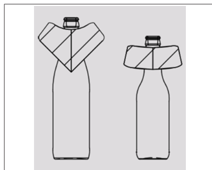
Рис. 31: Станиолевое кольцо на горлышко: ниже мундштука; перекрывается в зоне горлышка
