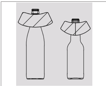
Рис. 24: Кольцевая этикетка на горлышко: перекрывается в зоне горлышка
