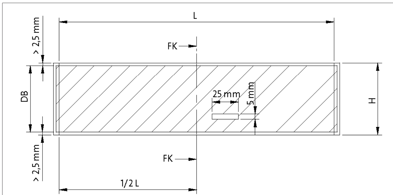
Рис. 110: Размеры этикеток
