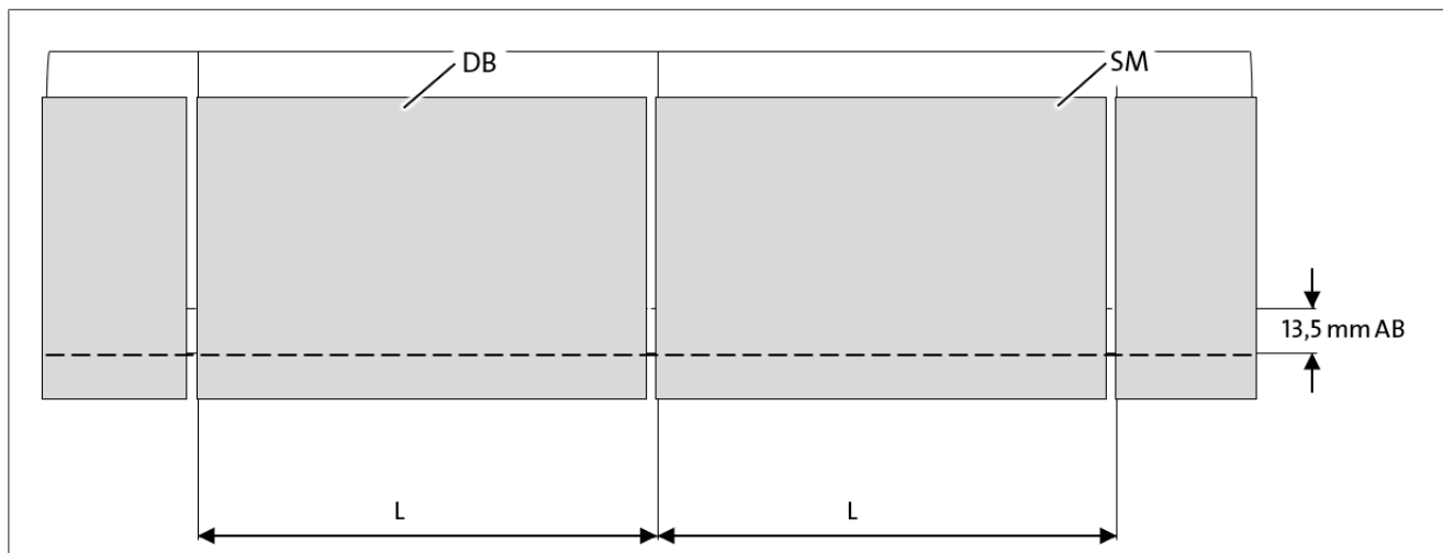
Рис. 86: Пример чертежа этикетки с прозрачной меткой отрезания
