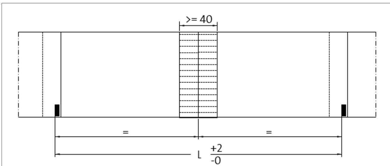
Рис. 72: Чертёж этикеток для склеивания этикеток на непрерывной ленте
