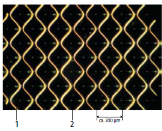
Рис. 12: Электромеханически гравированные углубления (максимальная глубина гравировки)
