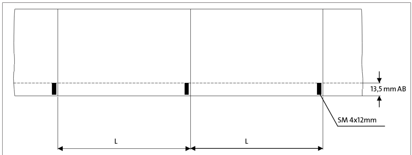
Рис. 74: Чертёж этикетки для управления меткой отрезания
