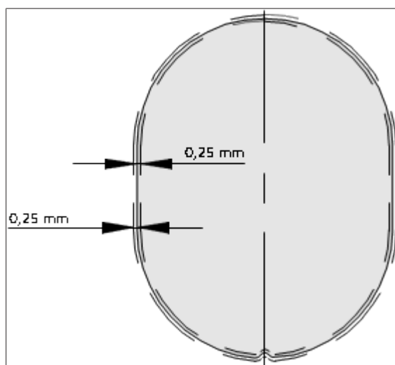
Рис. 54: Допуски на этикетки
