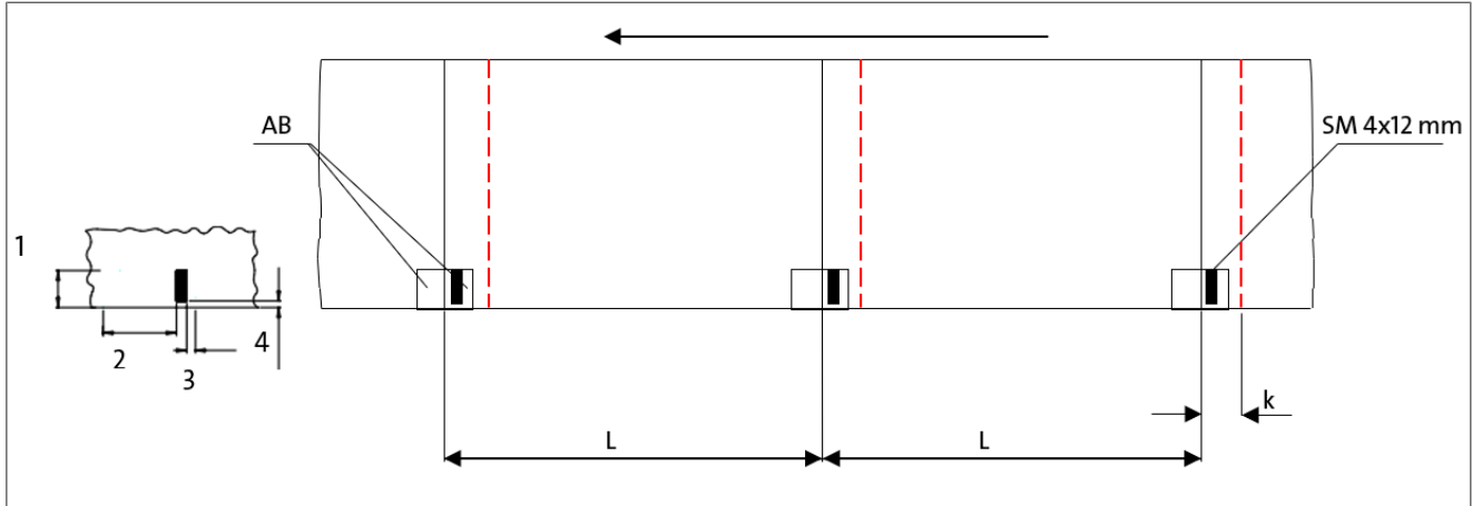
Рис. 75: Этикетка с зоной сканирования через окно
