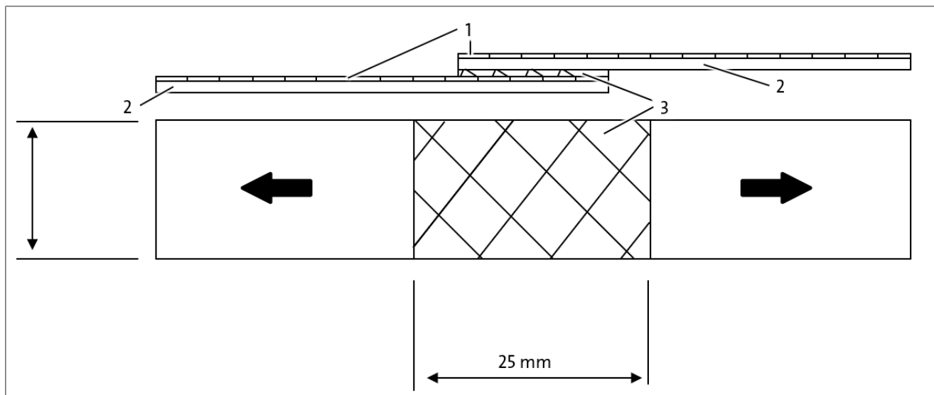
Рис. 106: Склеивание этикеток
