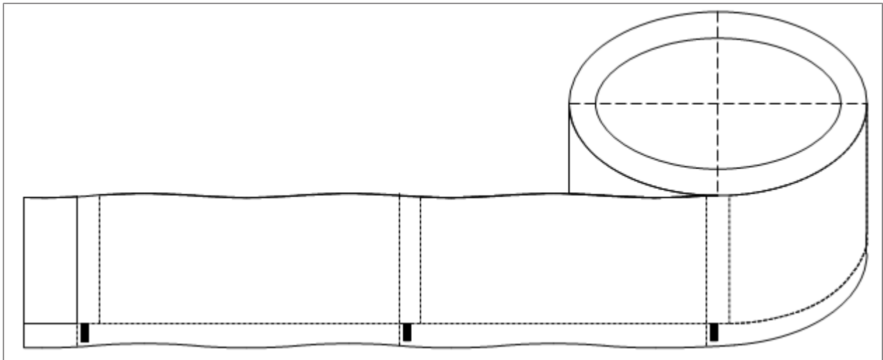
Fig. 64: Ejemplo de bordes de etiqueta ondulados
