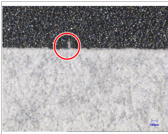
Fig. 107: Bordos de corte con flecos
