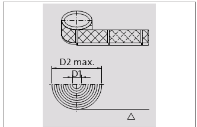
Fig. 69: Sentido de enrollado de la bobina para máquinas que marchan de derecha a izquierda
