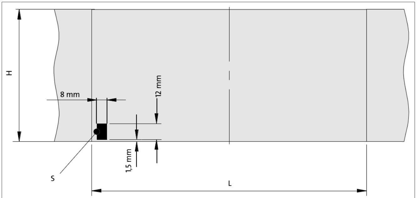
Fig. 95: Marca de corte luminiscente
