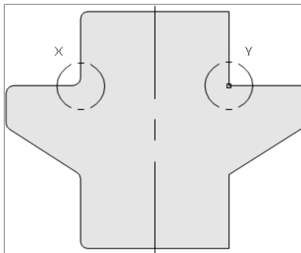
Fig. 51: Radios de vértices redondeados
