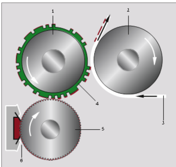
Fig. 8: Principio de la tipografía
