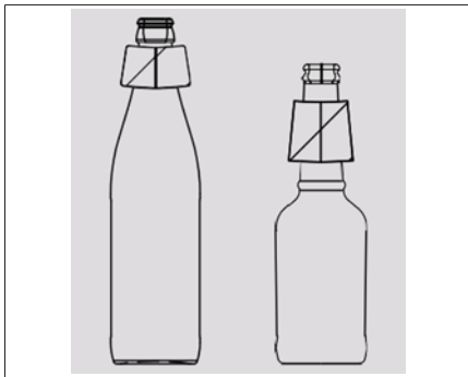
Fig. 23: Collarín: en la zona del cuello del envase
