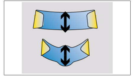
Fig. 50: Orientación errónea de las fibras
