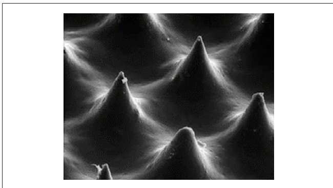
Fig. 9: Imagen microscópica de puntos de trama sobre una plancha flexográfica
