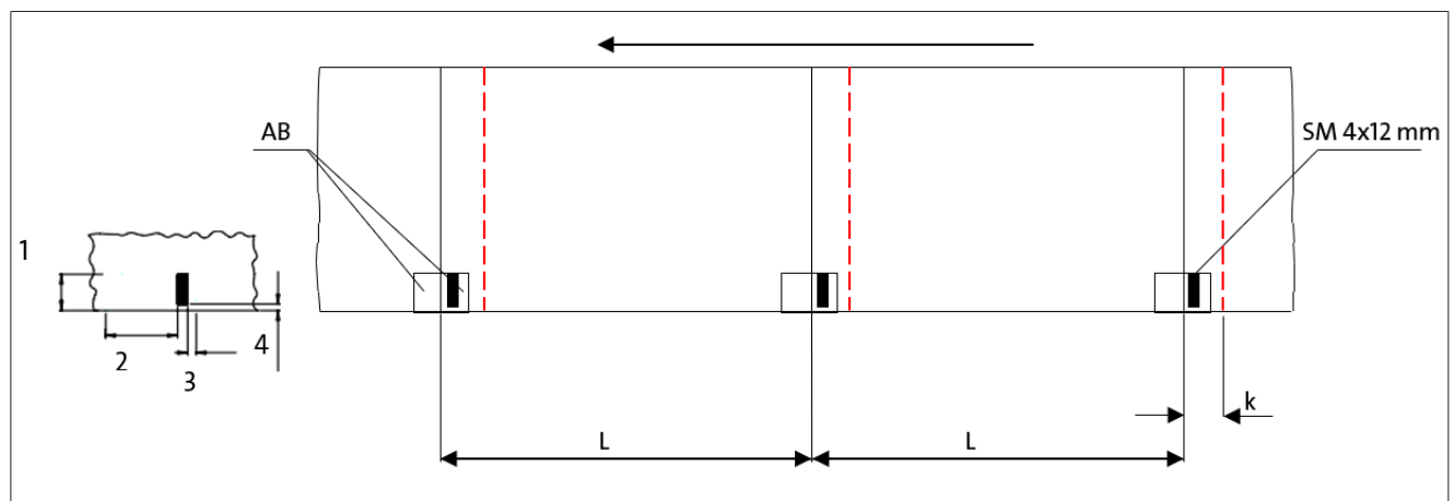
Fig. 75: Etiqueta con área de exploración definida por una ventana
