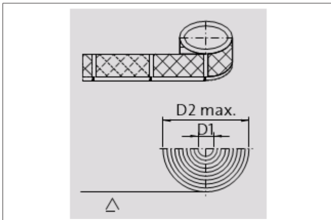
Fig. 68: Sentido de enrollado de la bobina para máquinas que marchan de izquierda a derecha
