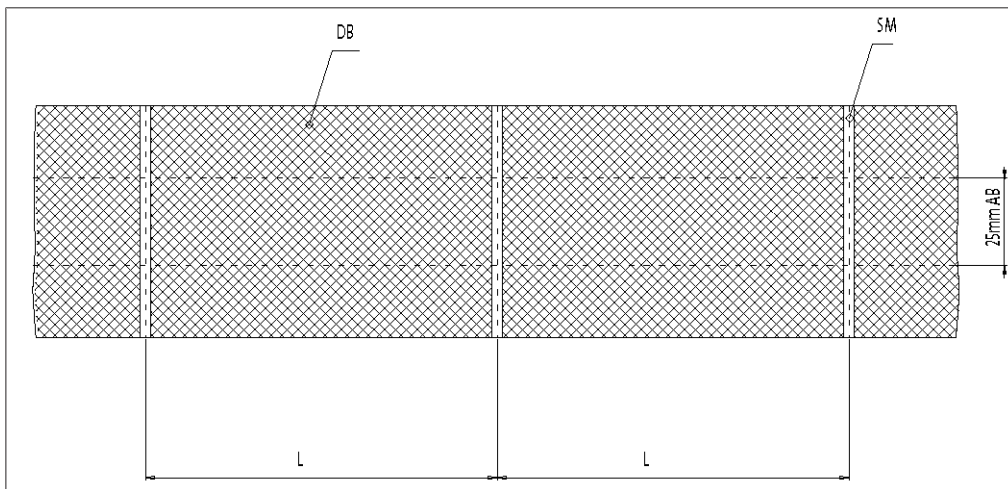
Fig. 121: Dibujo de etiqueta: geometría de las marcas de corte transparentes
