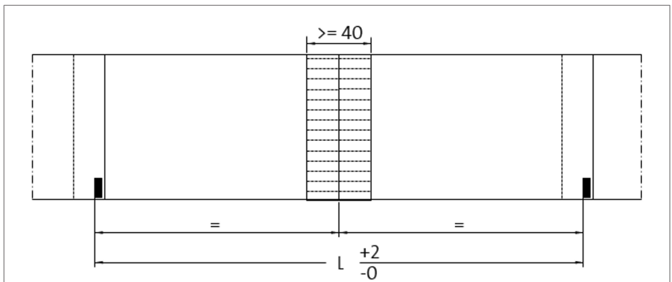
Fig. 72: Dibujo para el empalme de las etiquetas en bobina
