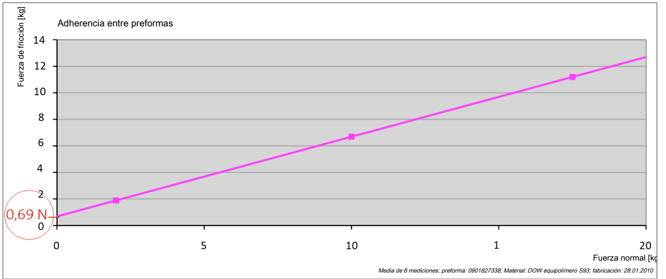
Fig. 130: Línea de la fuerza de adhesión respecto a la fuerza normal
