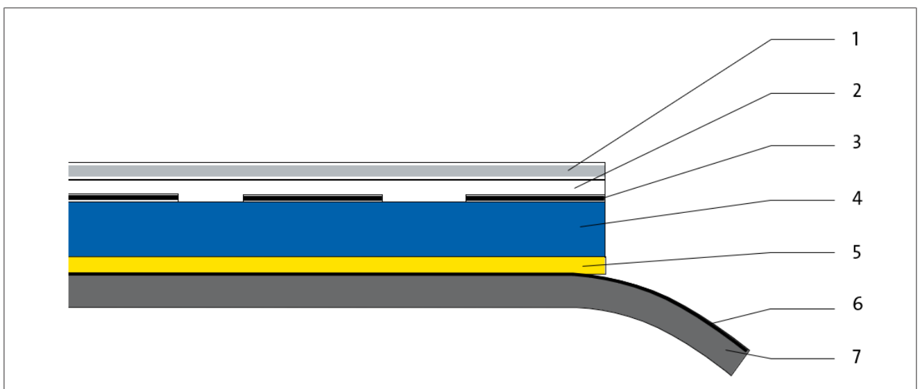
Fig. 105: Estructura del material
