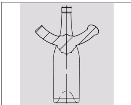
Fig. 29: Collarín de cava: especialmente para botellas de cava; se solapa en la zona del cuello/ de los hombros
