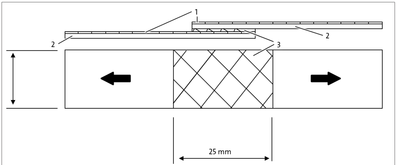
Fig. 106: Empalme de etiquetas
