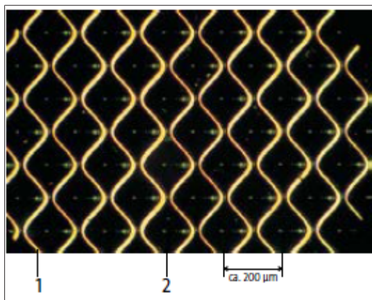
Fig. 12: Oquedades grabadas electromecánicamente (profundidad máxima de grabado)
