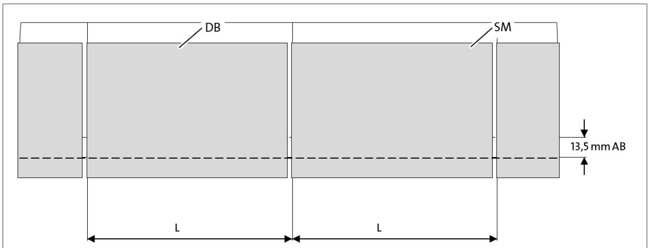
Fig. 86: Ejemplo de dibujo de etiqueta con marca de corte transparente
