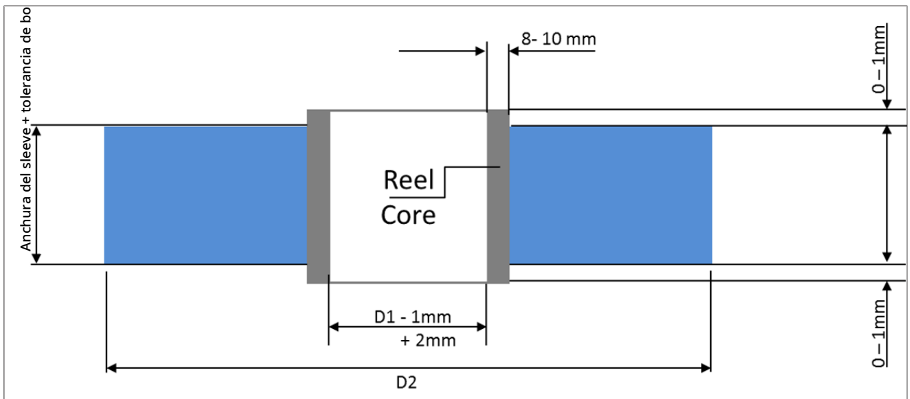
Fig. 127: Núcleo de bobina en etiquetas tipo sleeve
