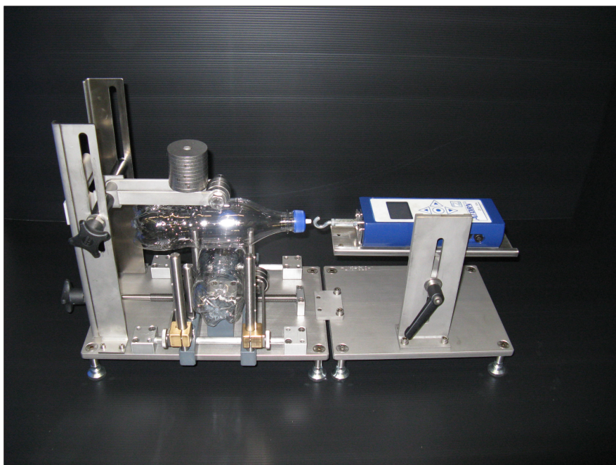
Fig. 128: Medidor de la adherencia entre envases
