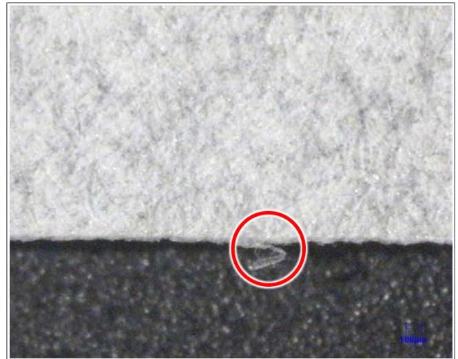
Fig. 66: Bordes de corte con flecos
