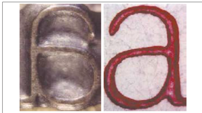
Fig. 10: Borde de engaste: característica distintiva de la flexografía
