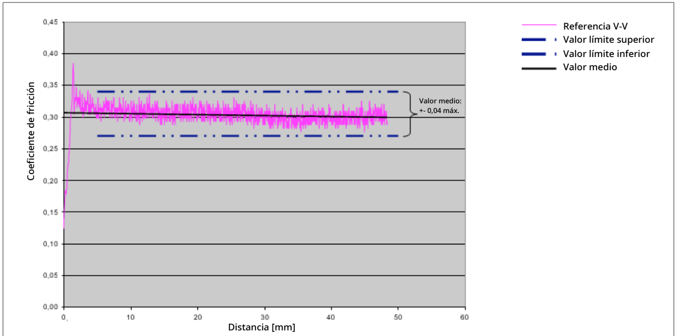
Fig. 60: Coeficiente de fricción de las etiquetas
