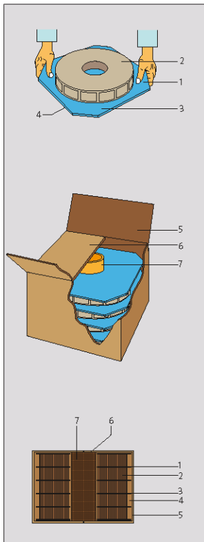
Fig. 2: Embalaje de bobinas de etiquetas
