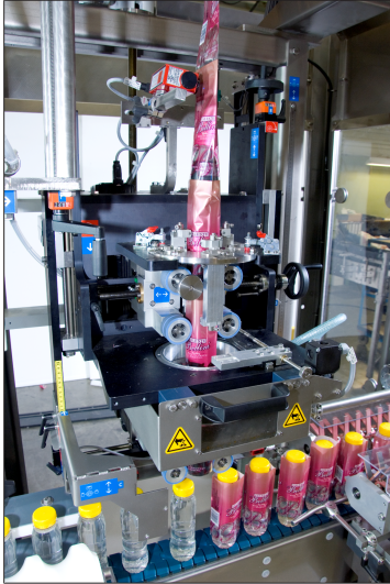
Fig. 114: Ejemplo de detección por sensor de la marca de corte
