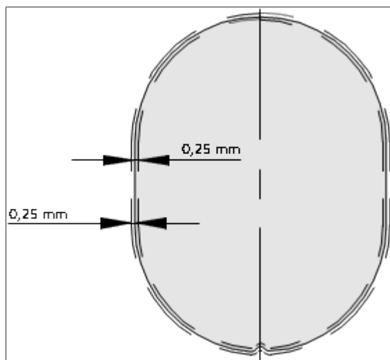
Fig. 54: Tolerancias de las etiquetas
